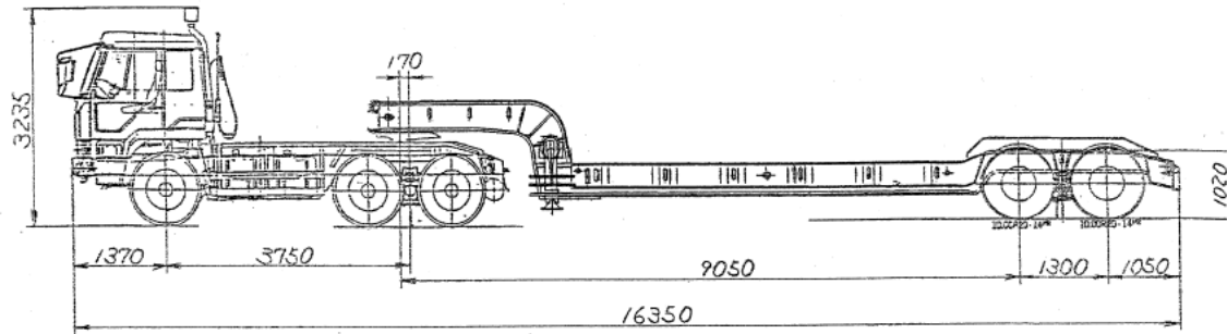
三菱BDGFV50JJR型トラクタ
