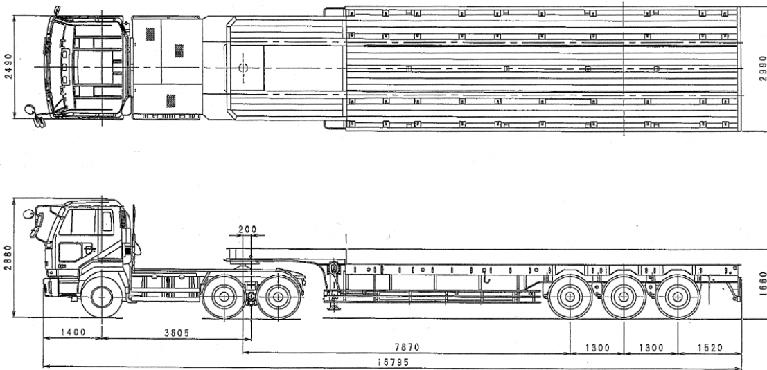
ニッサンディーゼルKL-CW632GHT型トラクタ 東急TL50J1C3S型セミトレーラ
