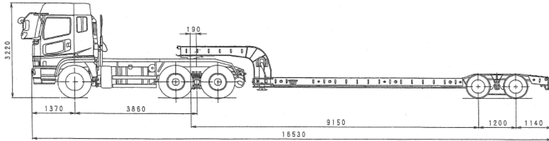
三菱QDG-FV50VJR型トラック
